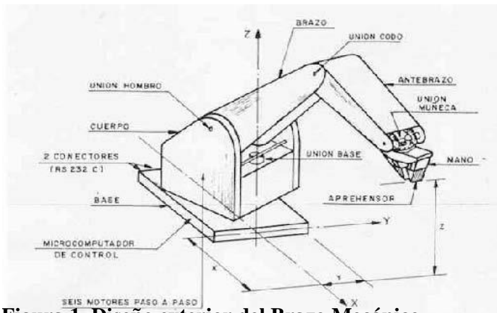
Figura 1. Diseño exterior del Brazo Mecánico
